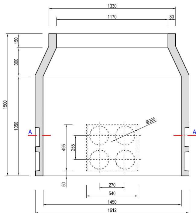
CORTE B-B
